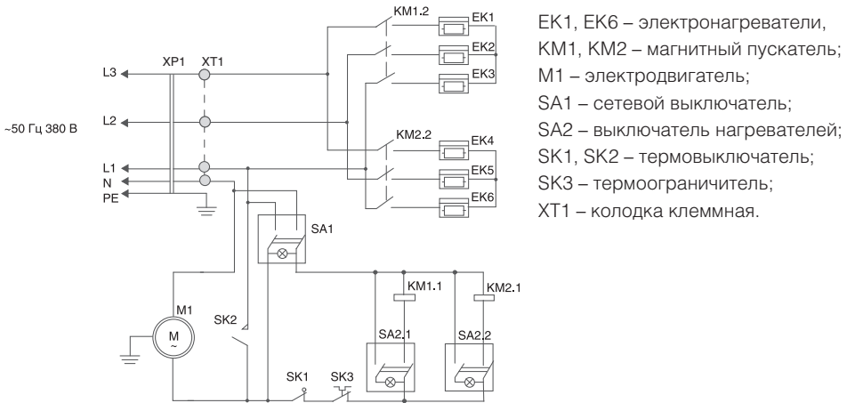
Рис. 4. Схема электрическая тепловентиляторов ВНР-15.000
