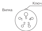
Рис. 5. Схема подключения контактов на вилку (ВНР-9.000, ВНР-15.000)
